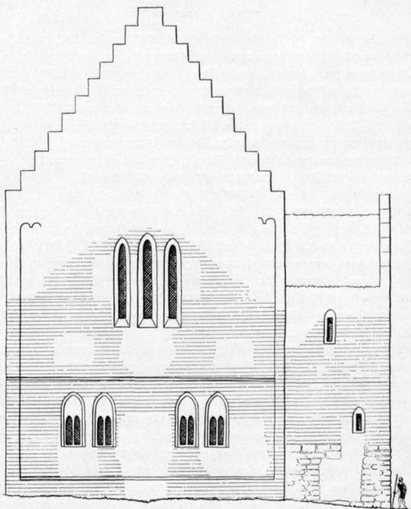
Fig. 2. Palatsets östfasad, preliminärt försök till rekonstruktion. Bevarade murpartier är streckade. Den övre fönsterggruppen i huvudbyggnaden (belägen i det förmodade kapellet) kan med säkerhet rekonstrueras. De två nedre är däremot spolierade så att någon säker bild av deras detaljer ej kan framställas. Ytterkonturerna är dock säkra. Sockeln är av kalksten och skråkantad. Språnget mellan de tjockare nedre och de tunnare övre delarna av själva gavelmurverket täckes också av en skråkantad kalkstenslist. — The east façade of the Palace, a preliminary attempt at reconstruction. The extant walls are hatched. The upper group of windows in the main building (situated in the conjectured Chapel) can be reconstructed with certainty, but the two lower ones are so badly damaged that no reliable representation of their details is possible. Their outer contours are certain, however. The socle of the wall is of limestone and chamfered. The projection between the thicker lower and the thinner upper parts of the actual gable masonry is also covered by a limestone chamfer.
