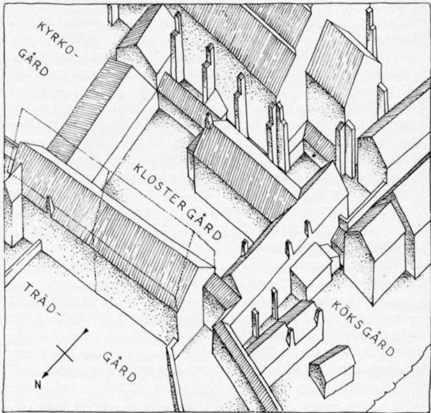
Fig. 1. Bilden avser att visa, dels var palatset, med sin saldel i väster och sin bostads(?)del i öster, är beläget i klosterkomplexet ävensom hur mycket av dess murhöjder som återstår, dels nunneklostrets byggnader så som de för närvarande kan preliminärt rekonstrueras. Bilden ersätter fig. 5 i uppsatsen »Gården Vastenis och klostret i Watzstena», Fornvännen 1958 h. 5—6. — This drawing is an attempt to show where the Palace with its Hall wing to the west and its residential(?)wing to the east is situated in the block of Convent buildings and also how much of its walls remain; also the Nunnery buildings at the present stage of their preliminary reconstruction. This drawing replaces Fig. 5 in the article on "The Manor of Vastenis and the Convent at Watzstena" in Fornvännen 1958, 5—6.
